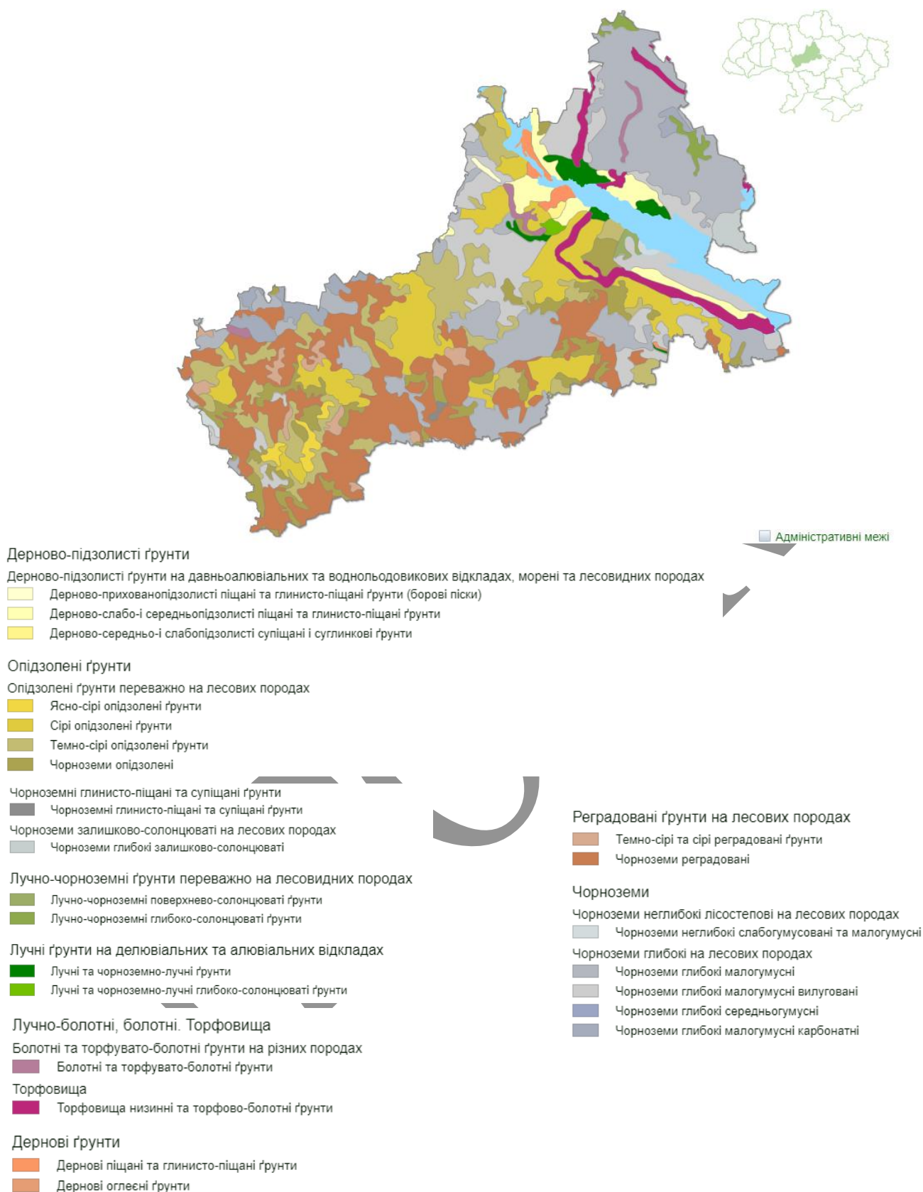
Рис. 5.1 Карта ґрунтів Черкаської області
