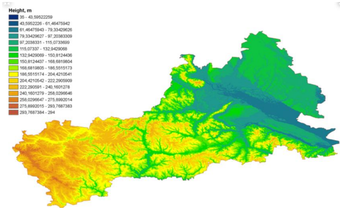
Рис. 3.1 Цифрова модель рельєфу Черкаської області
