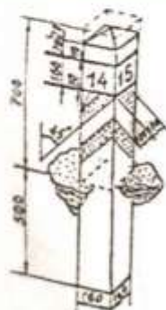
стовп залізобетонний
